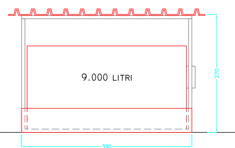
SERBATOIO GASOLIO CON BACINO E TETTOIA SCALA I: 50
