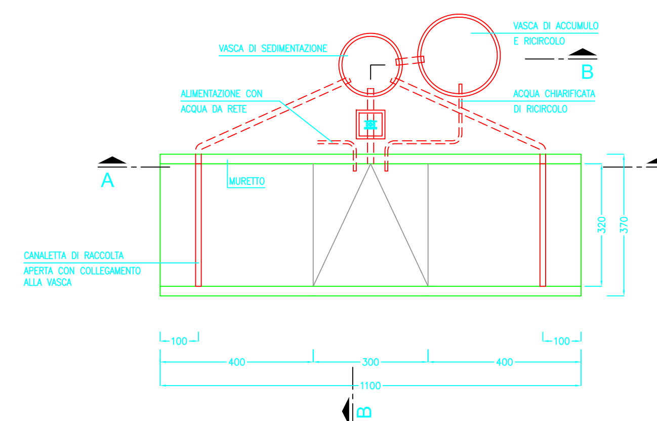
LAVARUOTE SCALA I: 100
