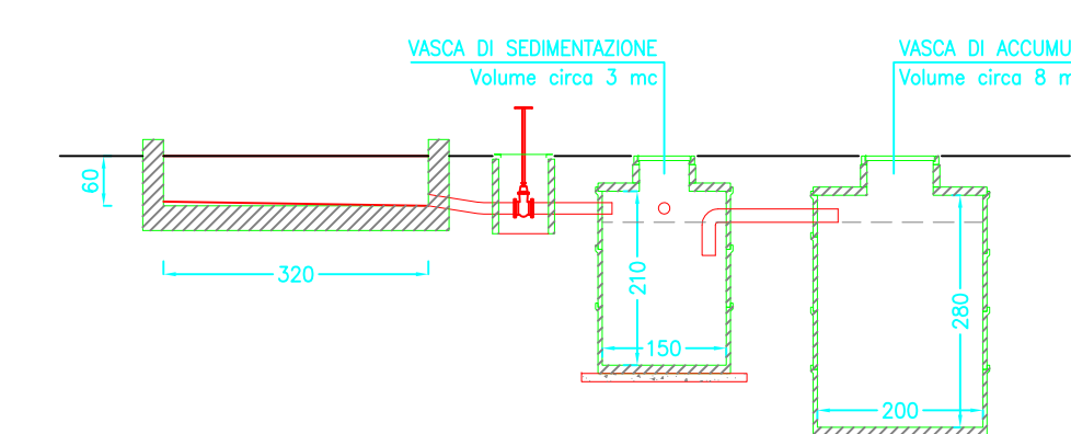
SEZIONE B-B
