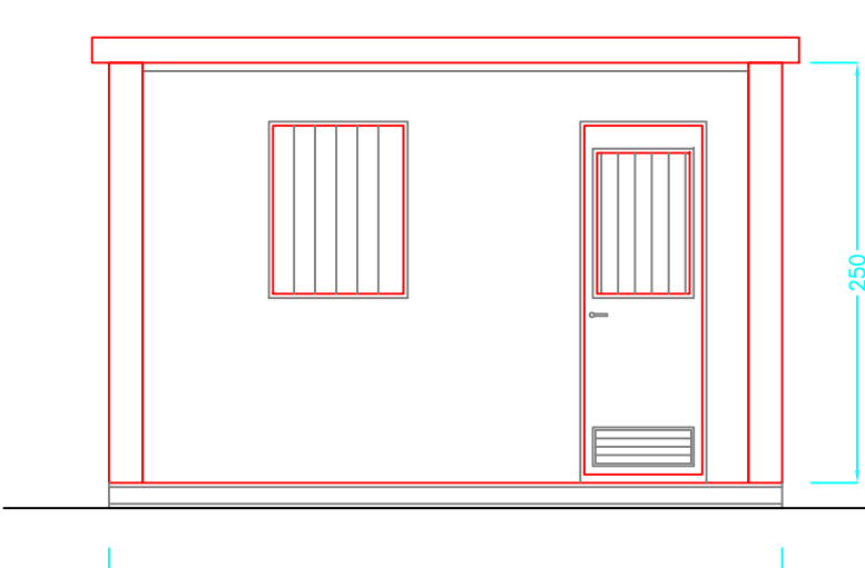
SPOGLIATOIO SCALA I: 50
